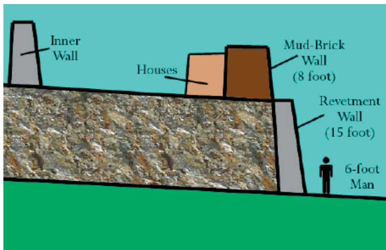
根據凱莎琳·肯揚的著作，耶利哥城牆結構（第四座城）的橫切面。
